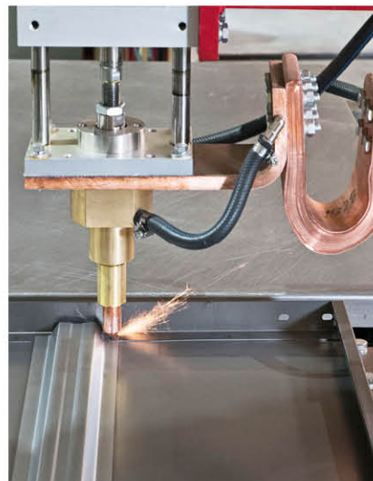
СВАРКА
